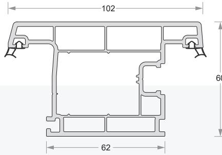
Casement Door Sash-Outward DP60-EL-655
