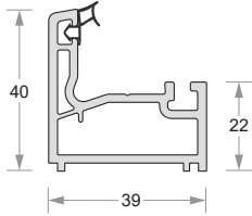
Casement Vent Frame DP39-VL-301
