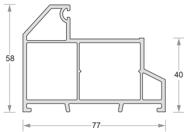
Door Frame DPDF7758
