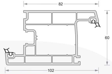
Casement Door Sash-Inward DP60-EL-656
