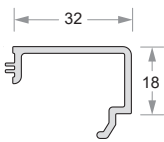
Louver Clip DP39-VL-305
