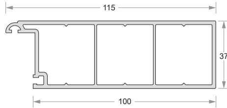
Door Sash DPDS11537
